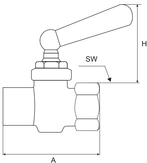
ברז למד לחץ עם ידית
